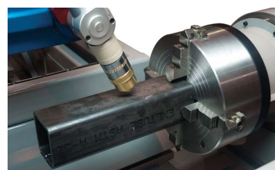
Corte rotatorio de tubos/tuberías
